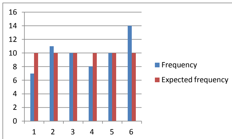
Fig. 3 Bar diagram sui dadi della Fig. 2
